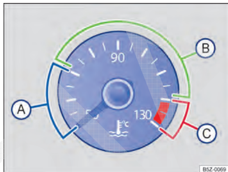
Fig. 130 Indicador de temperatura do líquido de arrefecimento do motor no instrumento combinado: (A) área fria; (B) área normal; (C) área de alerta.
