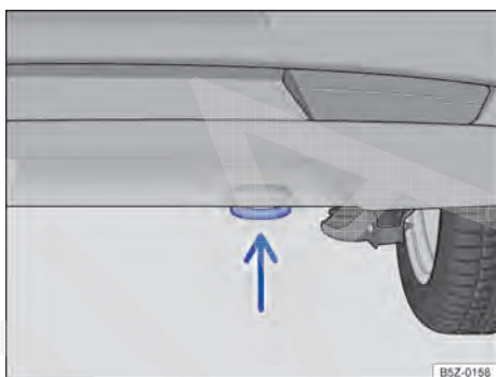
Fig. 188 No para-choque traseiro à direita: argola de reboque.
