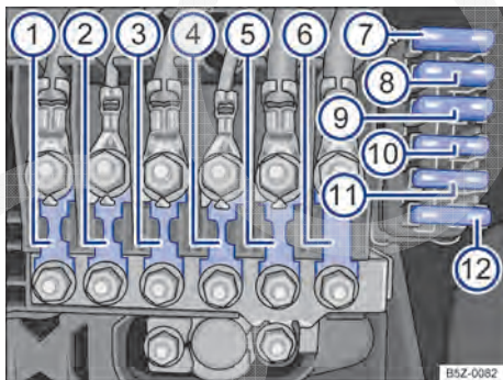
Fig. 170 Caixa de fusíveis.
