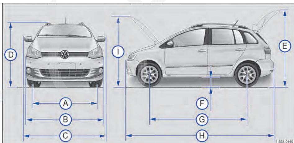
Fig. 192 Dimensões.
