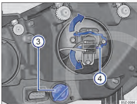
Fig. 172 No compartimento do motor: vista traseira do farol dianteiro direito sem cobertura de borracha: 3 indicadores de direção e 4 farol baixo.
