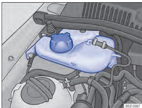
Fig. 133 No compartimento do motor: reservatório de gasolina para o sistema de partida a frio.
