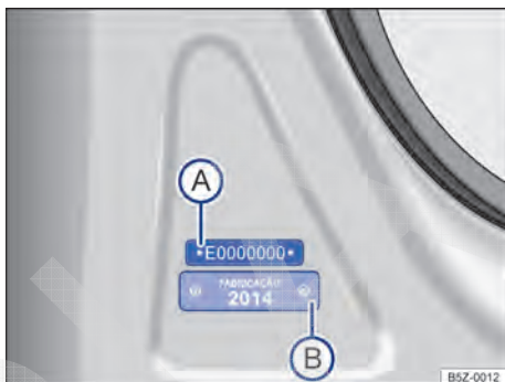
Fig. 190 Na coluna da porta dianteira direita: etiqueta com o número de identificação do veículo parcial (A) e etiqueta de identificação do ano de fabricação (B).
