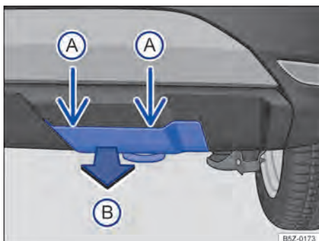
Fig. 189 No para-choque traseiro à direita: argola de reboque traseira - para-choque com cobertura removível. ▶
