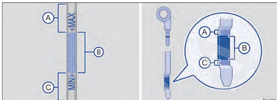
Fig. 128 Vareta de medição do óleo com marcas de nível do óleo do motor.
