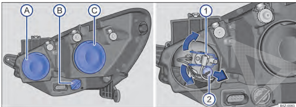
Fig. 171 No compartimento do motor: vista traseira do farol dianteiro direito com cobertura de borracha (esquerda): A farol alto e luz de posição, B indicadores de direção e C farol baixo. Vista traseira do farol dianteiro direito sem cobertura de borracha (direita): 1 farol alto, 2 luz de posição.
