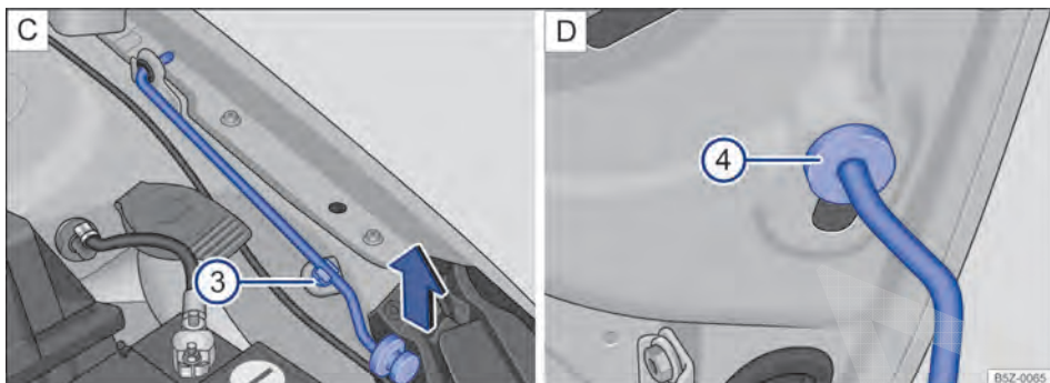
Fig. 127 C: haste de sustentação da tampa do compartimento do motor (3). D: tampa do motor protegida com a haste de sustentação da tampa (4).
