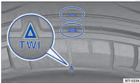
Fig. 142 Perfil do pneu: indicadores de desgaste.
