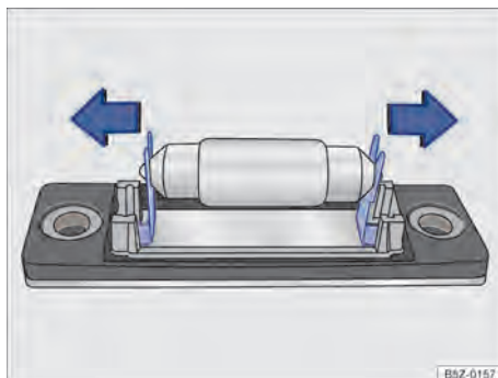
Fig. 184 Lanterna da placa de licença: remover a lâmpada.
