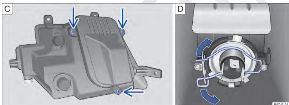
Fig. 178 No para-choque dianteiro: Ⓒ retirar os parafusos da cobertura da lâmpada e Ⓓ lâmpada do farol de neblina.
