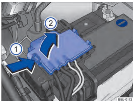
Fig. 185 Compartimento do motor: acesso ao terminal positivo da bateria.
