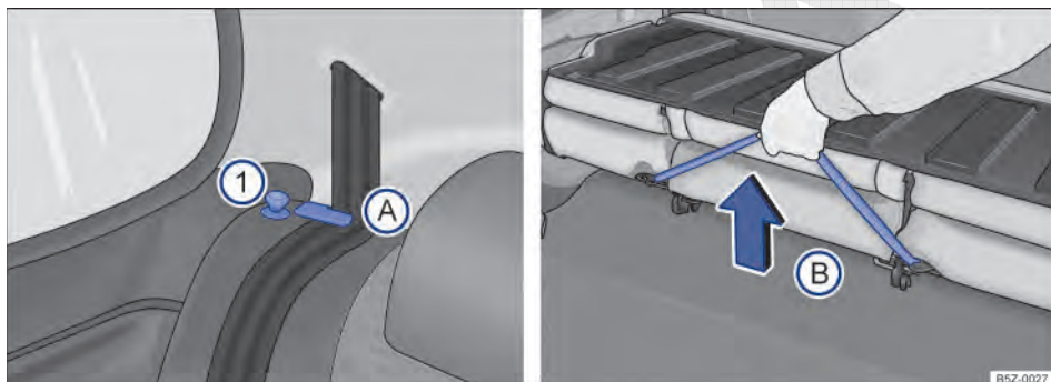
Fig. 74 Banco traseiro: pinos de desmontagem ①; posicionador para os caderços dos cintos (A); alça para desmontagem do conjunto do assoalho (B).
