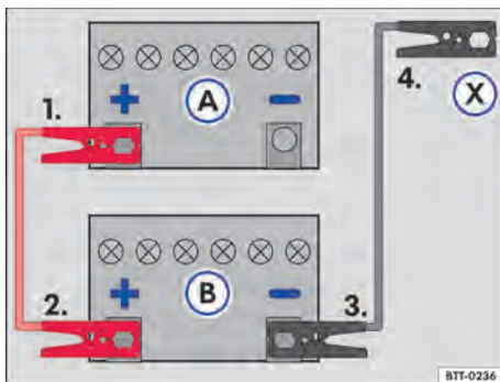
Fig. 186 Esquema para a conexão dos cabos auxiliares de partida: bateria do veículo descarregada (A) e bateria do veículo fornecedora de corrente (B).
