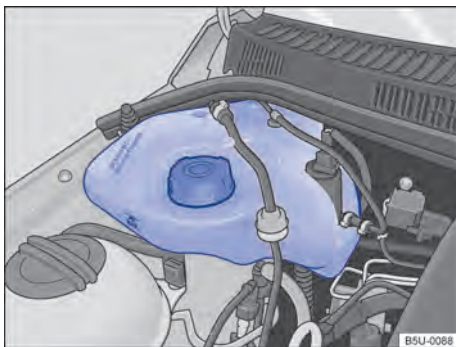
Fig. 209 No compartimento do motor: reservatório de gasolina para o sistema de partida a frio.
