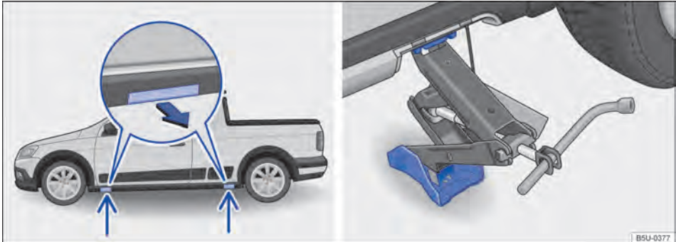
Fig. 222 Pontos de apoio do macaco e macaco posicionado no lado esquerdo traseiro do veículo - veículos com soleiras externas.
