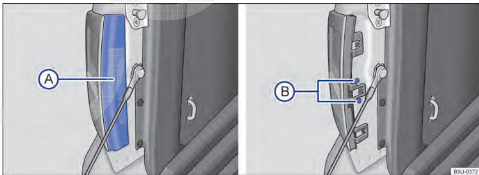
Fig. 169 No compartimento de carga: A desinstalar cobertura, B retirar os parafusos de fixação. ▶
