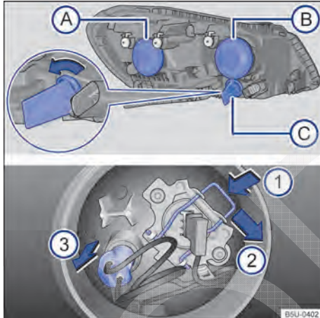
Fig. 165 Acesso à lâmpada incandescente do farol baixo.
