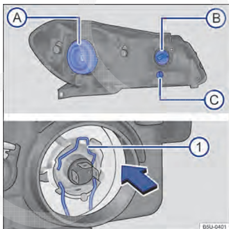
Fig. 162 No compartimento do motor: vista traseira do farol dianteiro com cobertura de borracha (lado esquerdo da ilustração) - A farol baixo / alto, B indicadores de direção e C luz de posição. Vista traseira do farol dianteiro sem a cobertura de borracha (lado direito da ilustração): 1 mola de travamento da lâmpada incandescente do farol baixo / alto.
