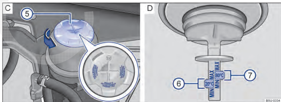
Fig. 110 No compartimento do motor (variante 2): C Reservatório do fluido da direção hidráulica. D Marcações para controle do nível do fluido da direção hidráulica.
