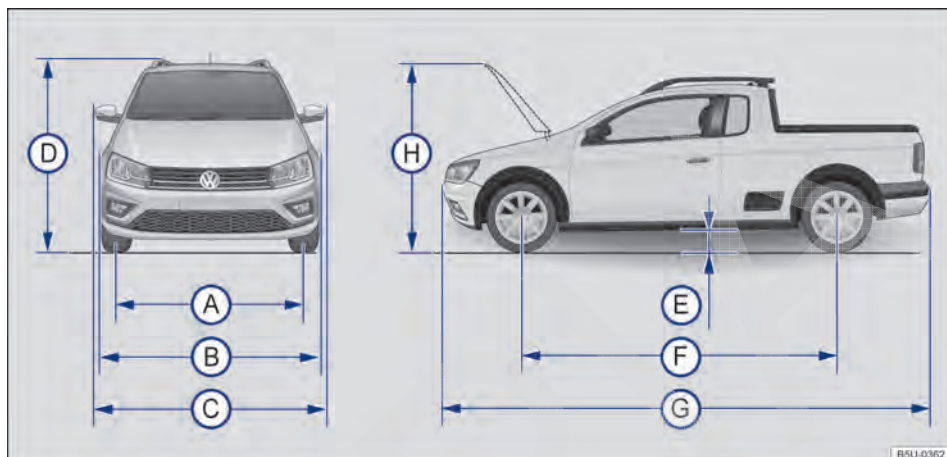
Fig. 215 Dimensões.
