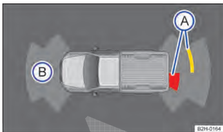
Fig. 117 Exibição do display do controle de distância de estacionamento (display colorido): A obstáculo reconhecido no segmento. B área examinada à frente do veículo.
