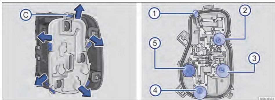
Fig. 170 Lanterna traseira: C desinstalar o suporte das lâmpadas e 1 , 2 , 3 , 4 e 5 desinstalar as lâmpadas.
