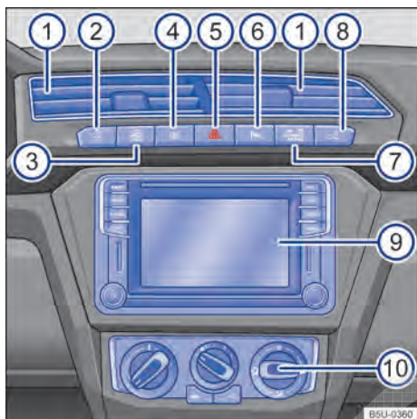
Fig. 32 Vista geral da parte superior do console central.
