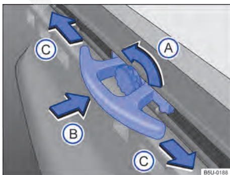
Fig. 149 No compartimento de carga: suporte deslizante para veículos com capota marítima.
