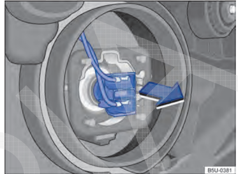
Fig. 165 Acesso à lâmpada incandescente do farol baixo.
