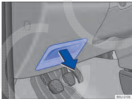
Fig. 175 No lado do condutor no painel de instrumentos: cobertura da caixa de fusíveis.
