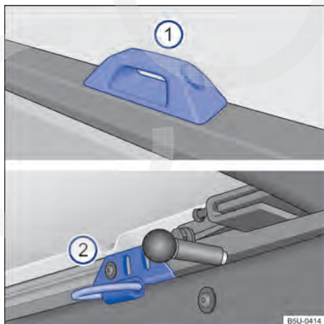
Fig. 147 No compartimento de carga: suportes fixos 1 para veículos sem capota marítima e 2 para veículos com capota marítima.
