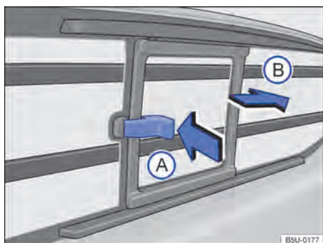
Fig. 74 No compartimento de carga: abertura do vidro corredeço.
