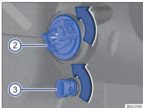
Fig. 163 No compartimento do motor: vista traseira do farol dianteiro 2 indicadores de direção e 3 luz de posição.
