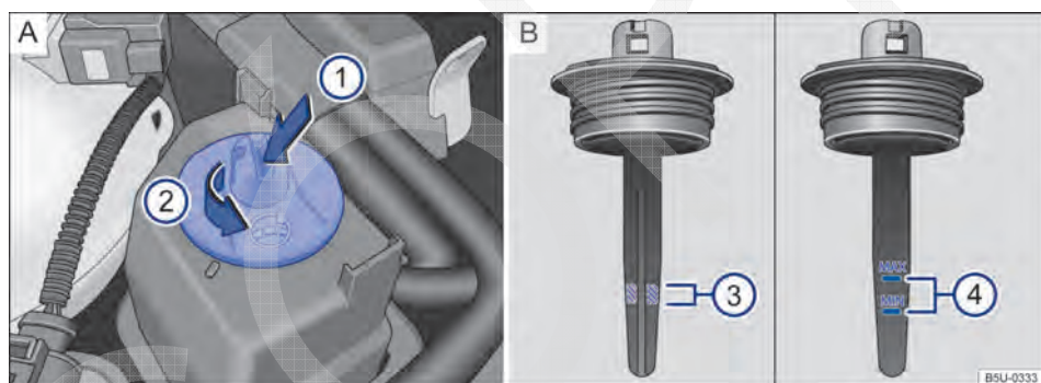
Fig. 109 No compartimento do motor (variante 1): A Reservatório do fluido da direção hidráulica. B Marcações para controle do nível do fluido da direção hidráulica.
