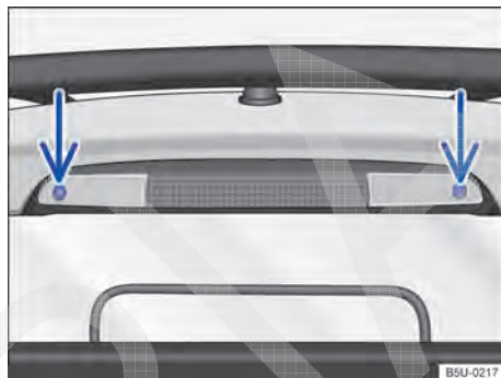
Fig. 173 No compartimento de carga: remover a lanterna de freio elevada.
