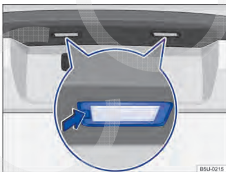
Fig. 171 No para-choque traseiro: remover a lanterna da placa de licença.
