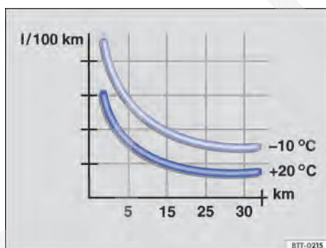
Fig. 105 Consumo de combustível em l/100 km em 2 temperaturas ambiente diferentes.
