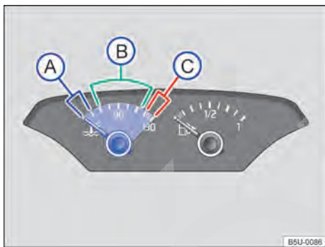
Fig. 48 Indicador de temperatura do líquido de arrefecimento do motor no instrumento combinado: (A) área fria; (B) área normal; (C) área de alerta.
