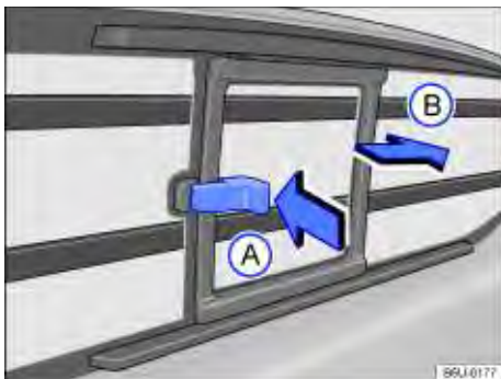
Fig. 38 No compartimento de carga: abertura do vidro corredeço.
