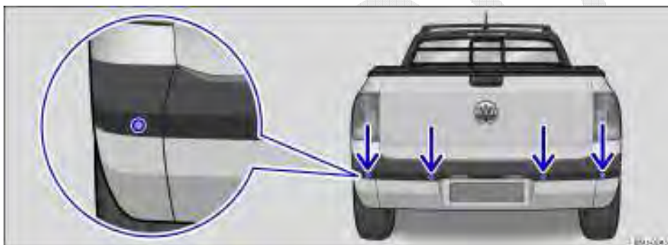
Fig. 118 Sensores de ultrassom do controle de distância de estacionamento no para-choque traseiro.
