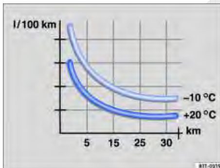
Fig. 114 Consumo de combustível em l/100 km em 2 temperaturas ambiente diferentes.
