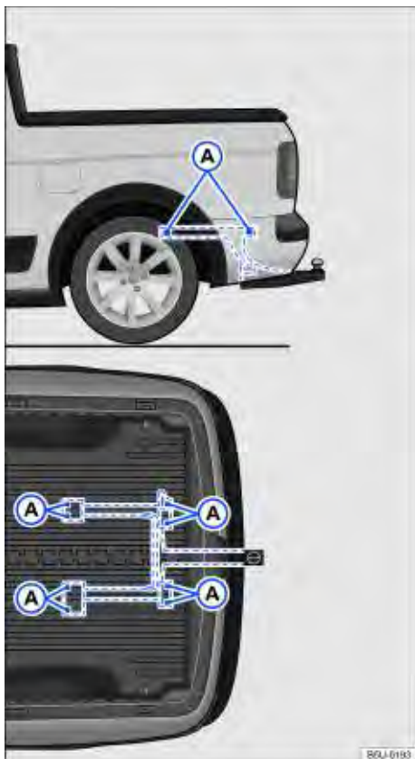
Fig. 87 Pontos de fixação para instalar um dispositivo de reboque posteriormente.
