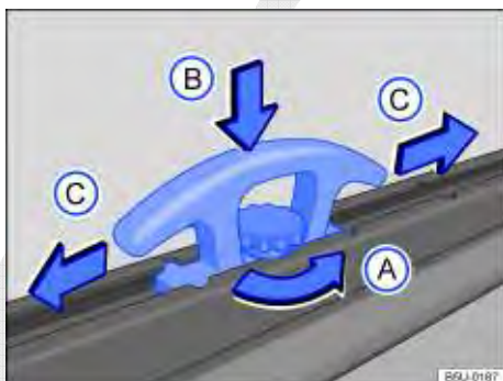
Fig. 82 No compartimento de carga: suporte deslizante para veículos sem capota marítima.
