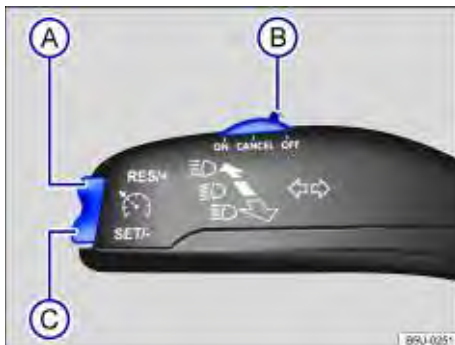
Fig. 121 À esquerda na coluna da direção: alavanca de operação do GRA.
