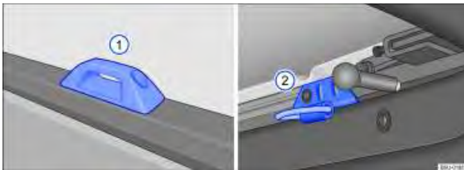
Fig. 81 No compartimento de carga: suportes fixos ① para veículos sem capota marítima e ② para veículos com capota marítima.
