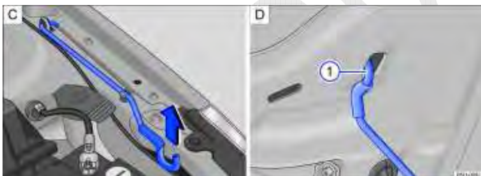
Fig. 129 (C) No compartimento do motor: haste de sustentação da tampa do compartimento do motor. (D) Tampa do compartimento do motor apoiada na haste de sustentação.
