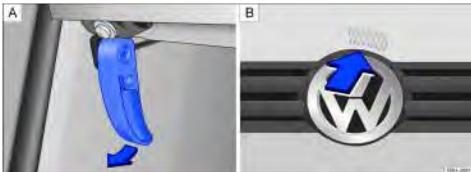
Fig. 128 (A) No espaço para os pés no lado do condutor: alavanca de desbloqueio da tampa do compartimento do motor. (B) Alavanca de destravamento para abrir a tampa do compartimento do motor.
