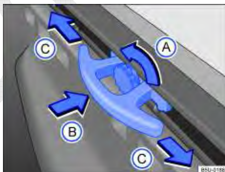
Fig. 83 No compartimento de carga: suporte deslizante para veículos com capota marítima.
