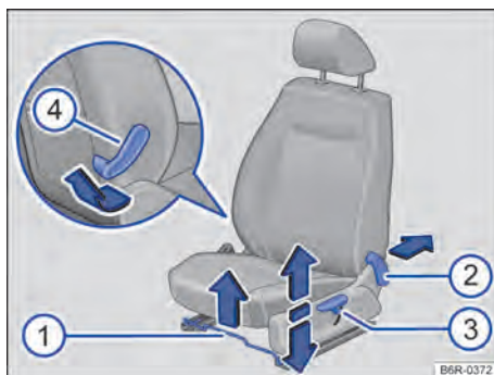
Fig. 63 No banco dianteiro: comandos.
