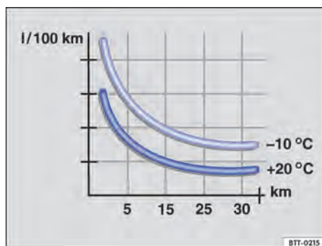
Fig. 86 Consumo de combustível em l/100 km em 2 temperaturas ambiente diferentes.
