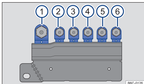
Fig. 141 No compartimento do motor em cima da bateria: disposição dos fusíveis.
