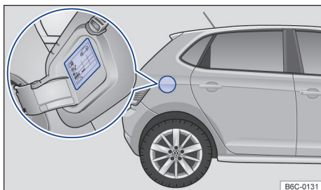
Fig. 158 Na parte interna da portinhola do tanque de combustível: etiqueta com a pressão dos pneus.
