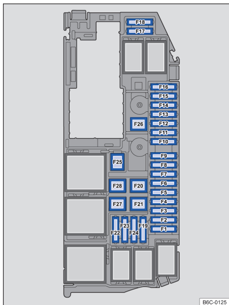
Fig. 140 No compartimento do motor: disposição dos fusíveis.
