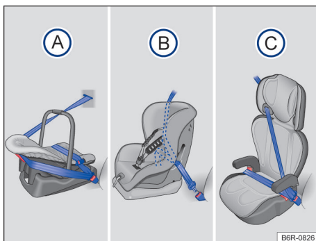
Fig. 43 As ilustrações (A), (B) e (C) mostram a fixação do sistema de retenção para crianças apenas com o cinto de segurança do veículo.
