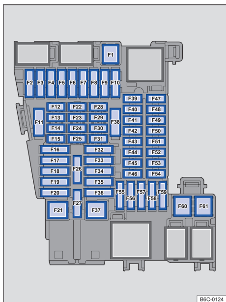
Fig. 138 No painel de instrumentos: disposição dos fusíveis.
