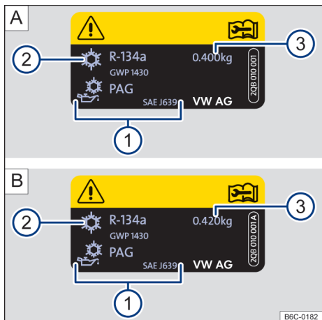
Fig. 172 A : informações do ar-condicionado - motor 1.0L. B : informações do ar-condicionado - motor 1.0L TSI e motor 1.6L.
