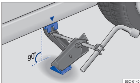
Fig. 166 Pontos de apoio do macaco e macaco posicionado no lado esquerdo traseiro do veículo.
