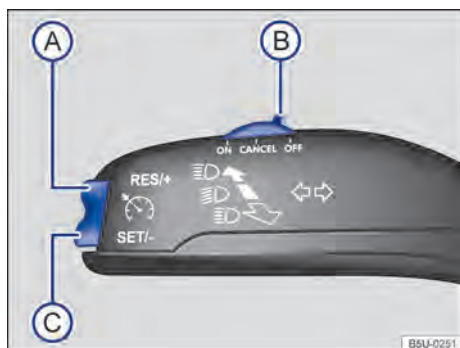
Fig. 113 À esquerda na coluna da direção: alavanca de operação do GRA.
