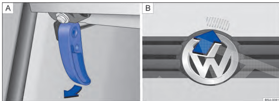
Fig. 121 A Alavanca de destravamento da tampa do compartimento do motor na área para os pés do lado do condutor. B Alavanca de destravamento na parte interna da tampa do compartimento do motor.
