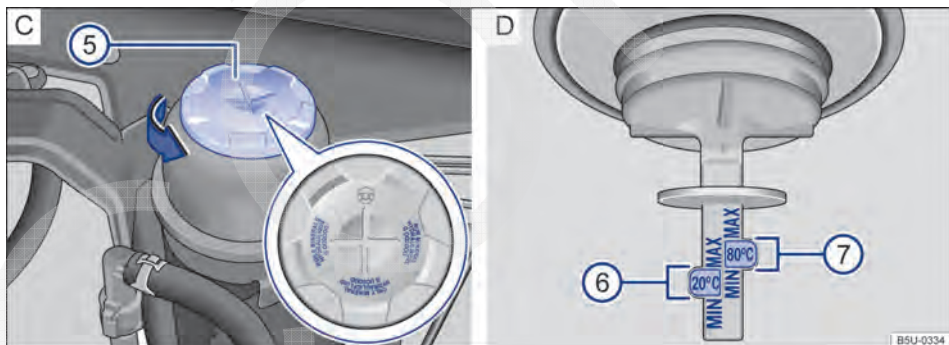
Fig. 108 No compartimento do motor (variante 2): C Reservatório do fluido da direção hidráulica. D Marcações para controle do nível do fluido da direção hidráulica.
