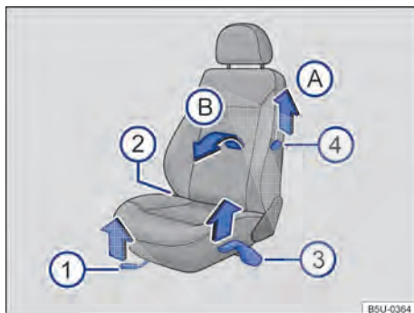
Fig. 34 Comandos do banco dianteiro esquerdo.
