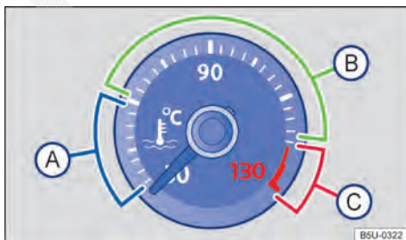
Fig. 126 Indicador de temperatura do líquido de arrefecimento do motor no instrumento combinado (variante 2): A) área fria; B) área normal; C) área de alerta.
