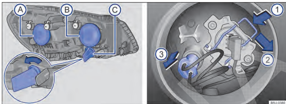
Fig. 171 No compartimento do motor: vista traseira do farol dianteiro com cobertura de borracha (lado esquerdo da ilustração) - (A) farol baixo, (B) farol alto e luz de posição, e (C) indicador de direção. Vista traseira do farol dianteiro sem a cobertura de borracha (lado direito da ilustração): ① mola de travamento da lâmpada incandescente do farol e ② luz de posição.
