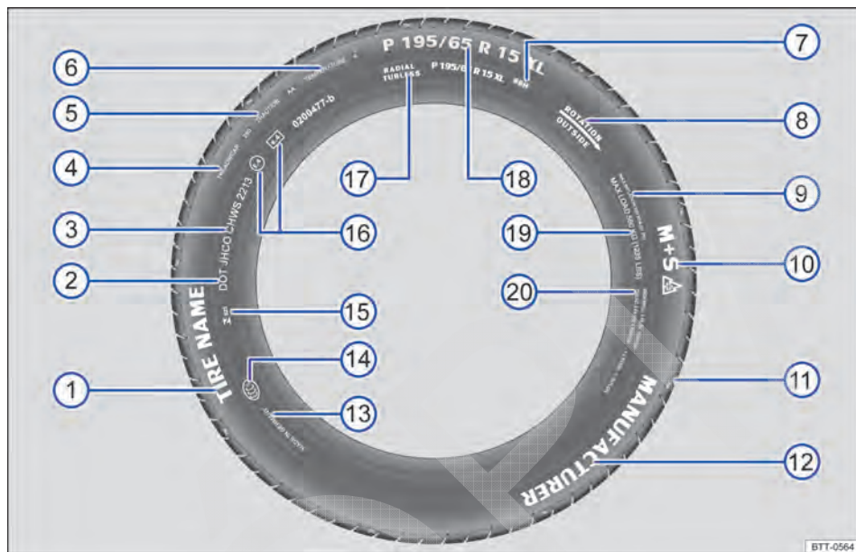
Fig. 136 Inscrição dos pneus internacional (exemplo).
