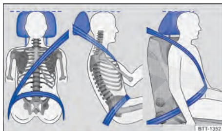
Fig. 49 Posição correta do cadarço do cinto de segurança e ajuste correto do apoio para cabeça.
