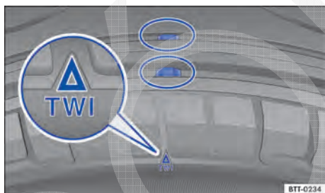
Fig. 134 Perfil do pneu: indicadores de desgaste.
