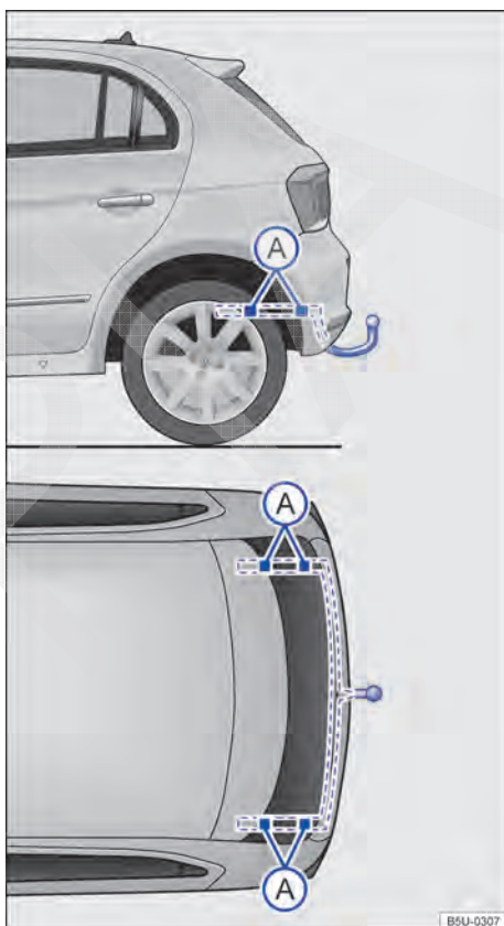
Fig. 76 Pontos de fixação para instalar um dispositivo de reboque posteriormente.
