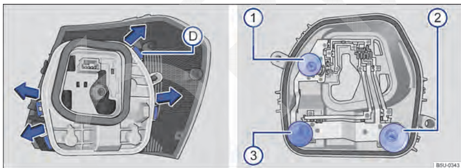
Fig. 175 Lanterna traseira: D desinstalar o suporte das lâmpadas e 1, 2 e 3 desinstalar as lâmpadas.
