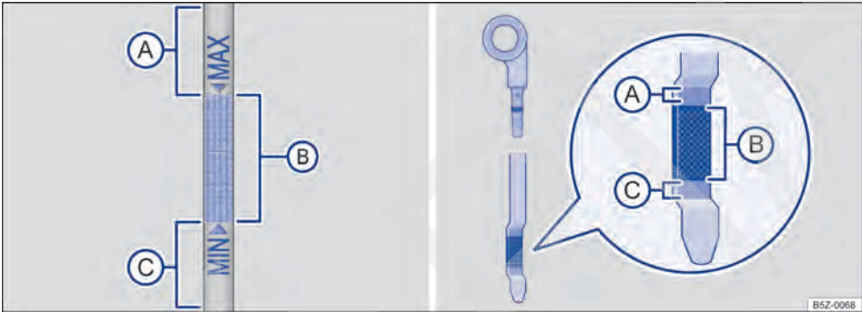
Fig. 123 Vareta de medição do óleo com marcas de nível do óleo do motor.
