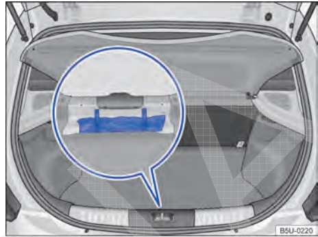
Fig. 155 No compartimento de bagagem: triângulo de segurança.
