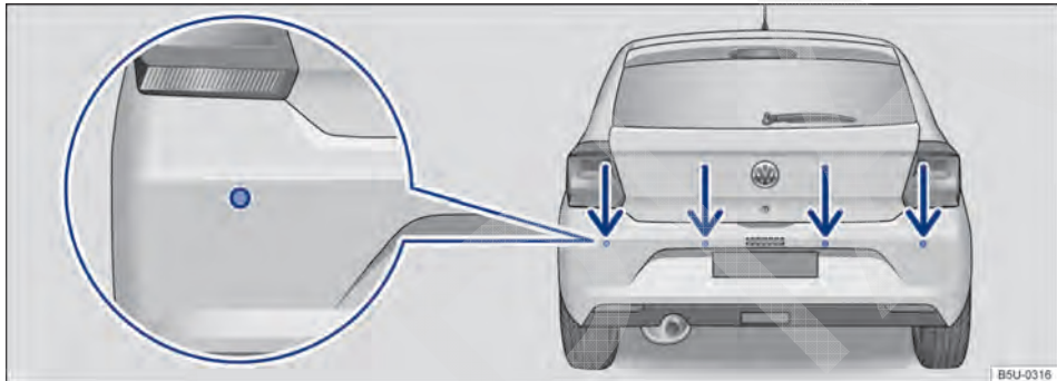
Fig. 109 Sensores de ultrassom do controle de distância de estacionamento no para-choque traseiro.
