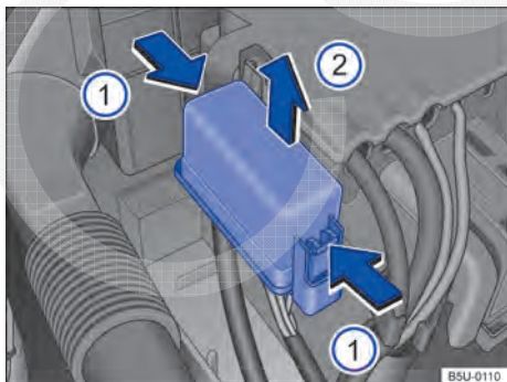
Fig. 164 No compartimento do motor: cobertura da caixa de fusíveis.
