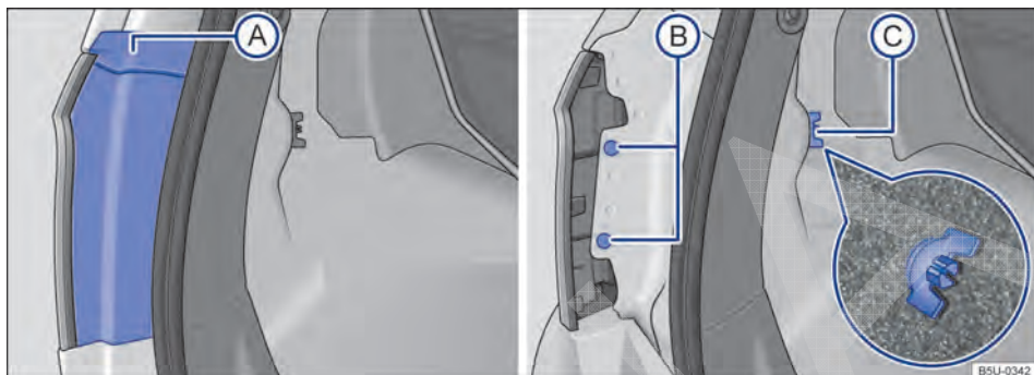
Fig. 174 No compartimento de bagagem: A desinstalar cobertura, B retirar os dois parafusos de fixação e C retirar o parafuso borboleta (lupa).
