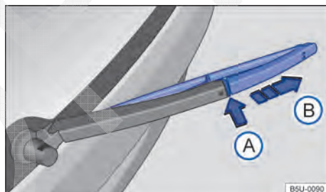
Fig. 144 Substituir a palheta do limpador do vidro traseiro.
