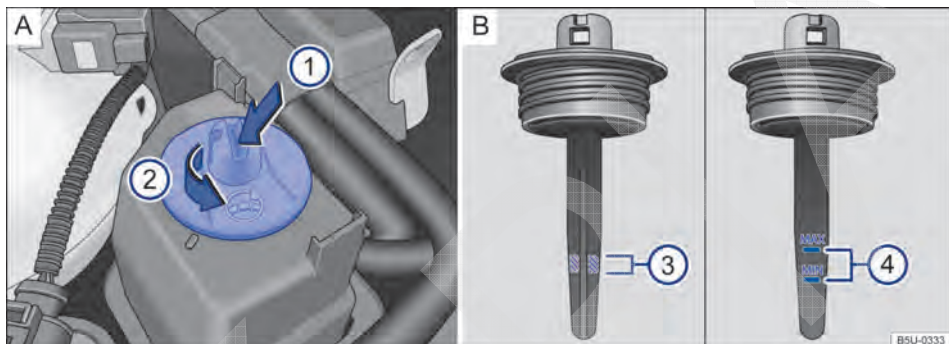
Fig. 107 No compartimento do motor (variante 1): A Reservatório do fluido da direção hidráulica. B Marcações para controle do nível do fluido da direção hidráulica.
