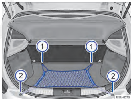
Fig. 75 No compartimento de bagagem: rede para bagagem.
