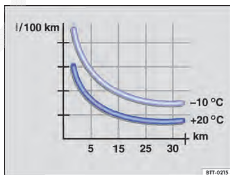
Fig. 106 Consumo de combustível em l/100 km em 2 temperaturas ambiente diferentes.
