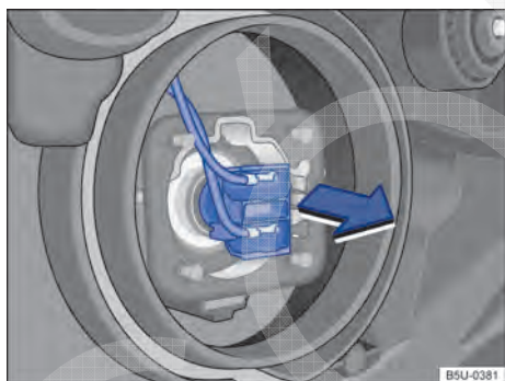
Fig. 172 Acesso à lâmpada incandescente do farol baixo.
