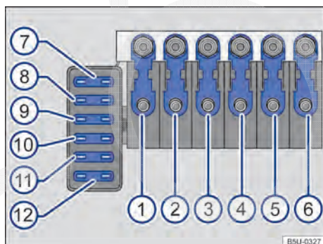
Fig. 168 Caixa de fusíveis.
