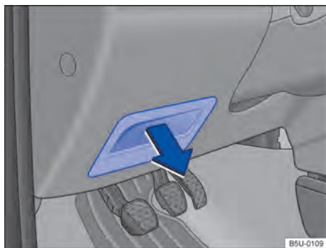
Fig. 184 No lado do condutor no painel de instrumentos: cobertura da caixa de fusíveis.
