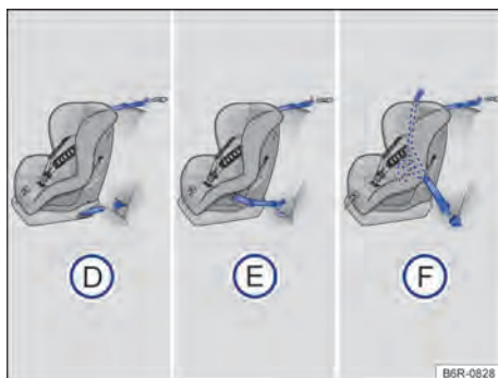
Fig. 36 No banco traseiro: as figuras D e E mostram o princípio da fixação do sistema de retenção para crianças nos olhais de retenção inferiores e com o cinto de fixação superior. A figura F mostra a fixação do sistema de retenção para crianças com o cinto de segurança do veículo e com o cinto de fixação superior.
