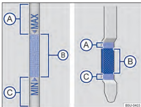
Fig. 195 Vareta de medição do óleo com marcas de nível do óleo do motor.
