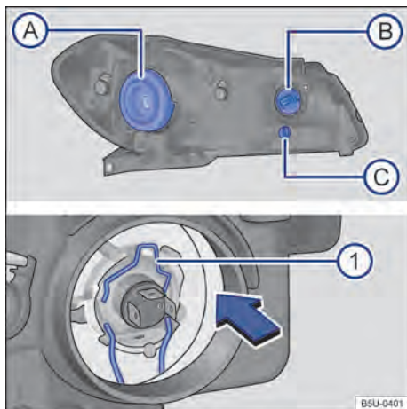
Fig. 175 No compartimento do motor: vista traseira do farol dianteiro com cobertura de borracha (lado esquerdo da ilustração) - (A) farol baixo / alto, (B) indicadores de direção e (C) luz de posição. Vista traseira do farol dianteiro sem a cobertura de borracha (lado direito da ilustração): (1) mola de travamento da lâmpada incandescente do farol baixo / alto. ▶
