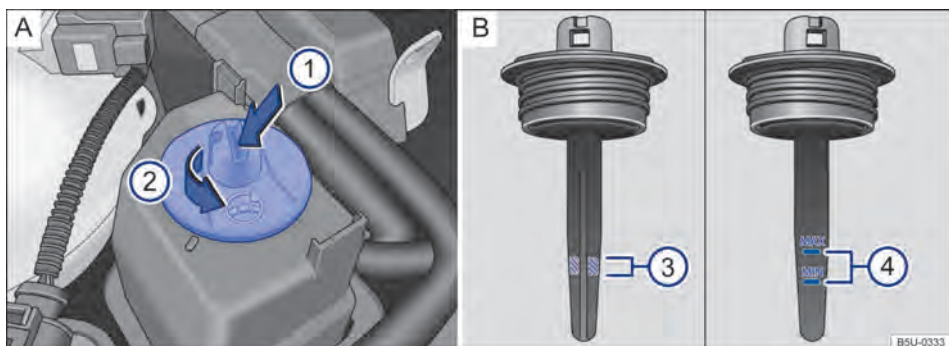
Fig. 87 No compartimento do motor (variante 1): A Reservatório do fluido da direção hidráulica. B Marcações para controle do nível do fluido da direção hidráulica.
