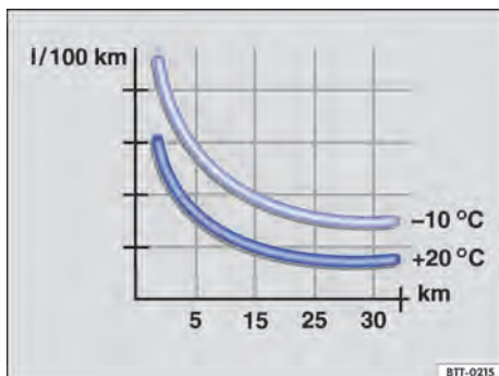
Fig. 79 Consumo de combustível em l/100 km em 2 temperaturas ambiente diferentes.
