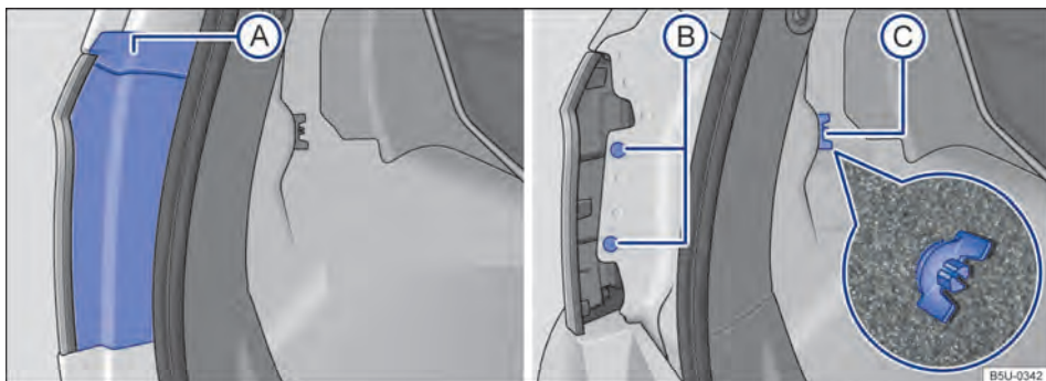
Fig. 180 No compartimento de bagagem: A desinstalar cobertura, B retirar os dois parafusos de fixação e C retirar o parafuso borboleta (lupa).
