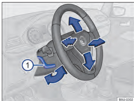
Fig. 53 Embaixo e a esquerda do volante junto com o revestimento da coluna de direção: alavanca de ajuste da posição do volante.
