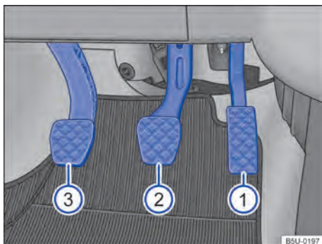
Fig. 75 Na área para os pés: pedais em veículos com transmissão manual.
