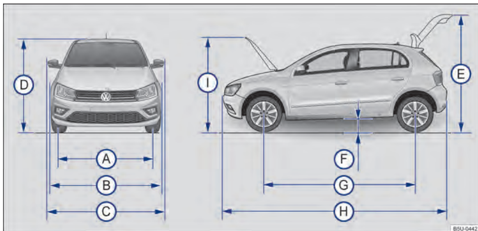
Fig. 219 Dimensões.
