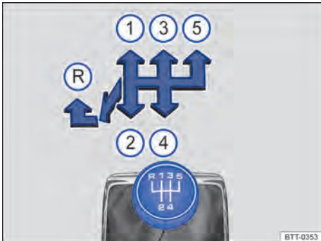
Fig. 82 Esquema de troca de marchas da transmissão manual de 5 marchas.
