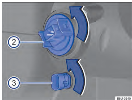
Fig. 176 No compartimento do motor: vista traseira do farol dianteiro ② indicadores de direção e ③ luz de posição.
