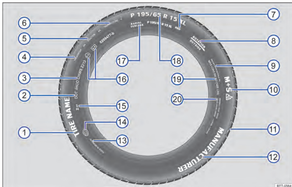
Fig. 207 Inscrição dos pneus internacional (exemplo).
