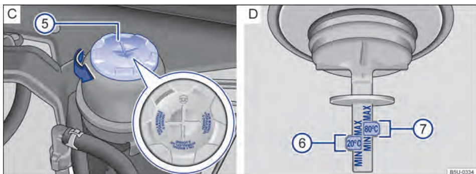
Fig. 88 No compartimento do motor (variante 2): C Reservatório do fluido da direção hidráulica. D Marcações para controle do nível do fluido da direção hidráulica.
