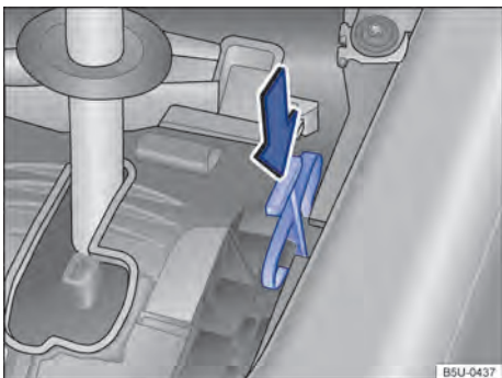
Fig. 86 Desinstalar a cobertura da alavanca seletora e destravar o bloqueio da alavanca seletora emergencialmente.
