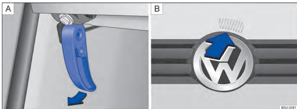
Fig. 192 [A] Alavanca de destravamento da tampa do compartimento do motor na área para os pés do lado do condutor. [B] Alavanca de destravamento na parte interna da tampa do compartimento do motor.
