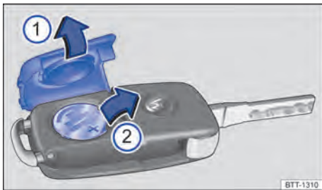
Fig. 46 Chave do veículo com comando remoto: ① Abrir a tampa do alojamento da bateria. ② Remover a bateria.
