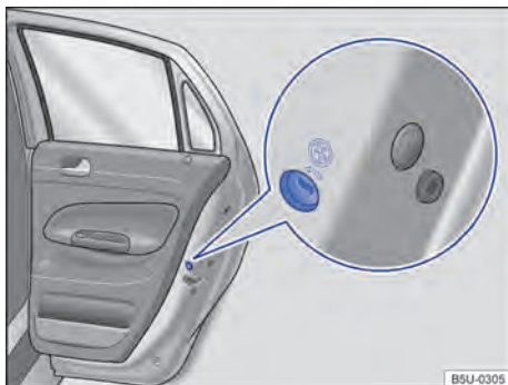
Fig. 40 Na porta traseira (lado direito): localização da trava de segurança para crianças.
