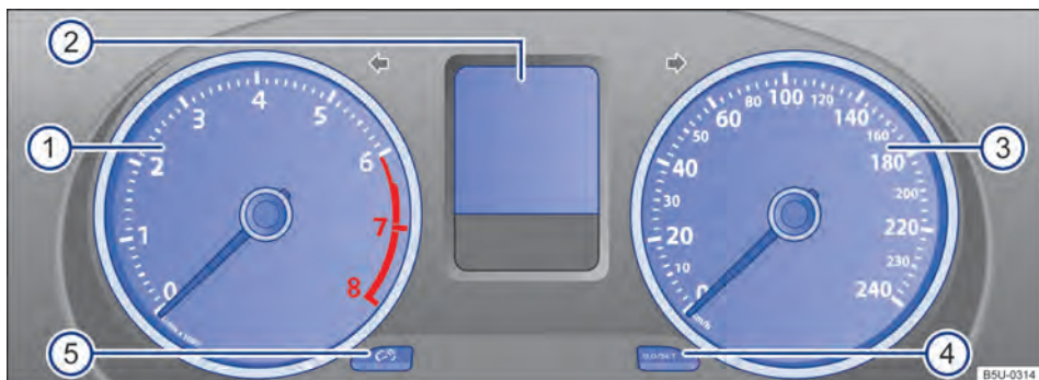
Fig. 11 Instrumento combinado no painel de instrumentos (variante 1).
