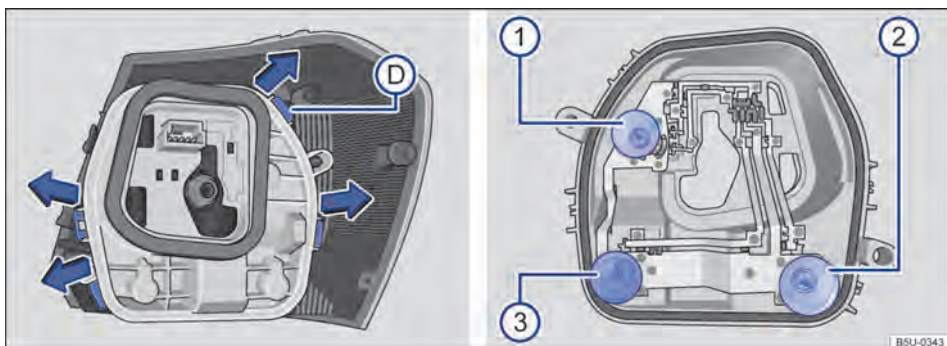
Fig. 181 Lanterna traseira: D desinstalar o suporte das lâmpadas e 1 , 2 e 3 desinstalar as lâmpadas.
