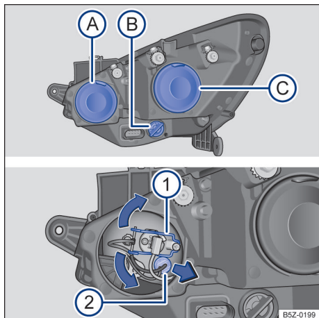
Fig. 118 No compartimento do motor: vista traseira do farol dianteiro direito com cobertura de borracha (esquerda): A farol alto e luz de posição, B indicadores de direção e C farol baixo. Vista traseira do farol dianteiro direito sem cobertura de borracha (direita): 1 farol alto, 2 luz de posição.
