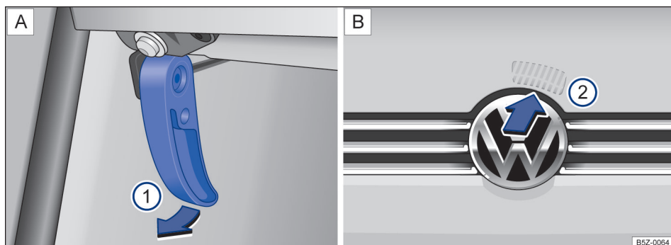
Fig. 142 A: alavanca de destravamento na área para os pés do lado do condutor ①. B: alavanca de destravamento na parte interna da tampa do compartimento do motor ②.
