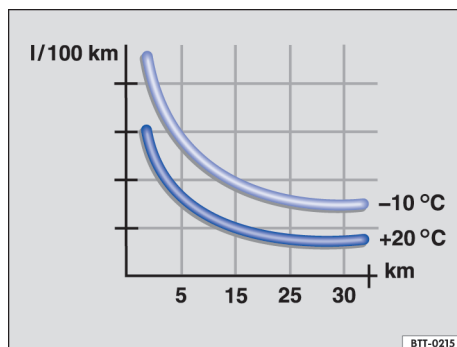
Fig. 83 Consumo de combustível em I/100 km em 2 temperaturas ambiente diferentes.
