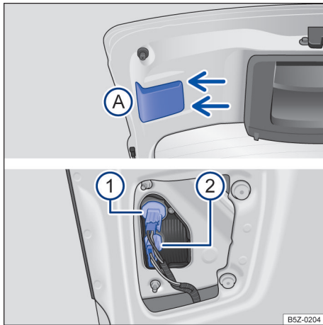
Fig. 125 Lanterna traseira: (A) desinstalar a cobertura e ① e ② desinstalar as lâmpadas.
