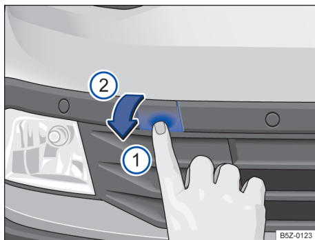
Fig. 138 No para-choque dianteiro à direita: soltar e remover a cobertura.
