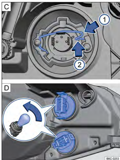
Fig. 167 No compartimento do motor: cobertura do indicador de direção do farol alto e baixo.
