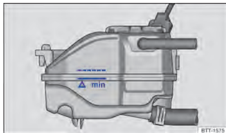
Fig. 187 No compartimento do motor: marcação no reservatório de expansão do líquido de arrefecimento do motor.
