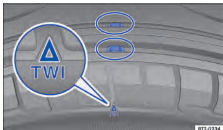
Fig. 195 Perfil do pneu: indicadores de desgaste.
