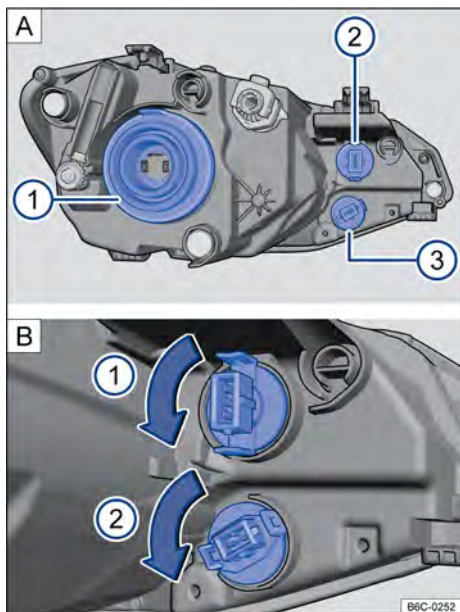
Fig. 166 No compartimento do motor: farol dianteiro. ① Luz de rodagem diurna e luz de posição e ② Indicadora de direção.
