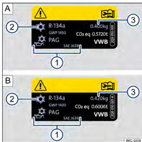
Fig. 208 A): informações do ar-condicionado - motor 1.0L. B): informações do ar-condicionado - motor 1.0L TSI, motor 1.4L TSI e motor 1.6L.
