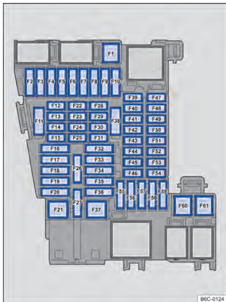
Fig. 173 No painel de instrumentos: disposição dos fusíveis.
