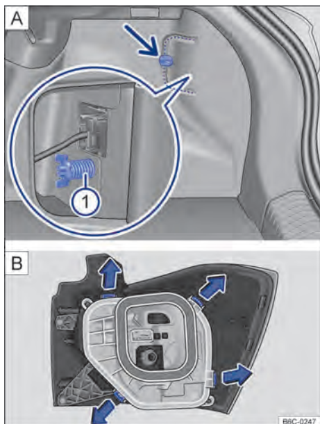
Fig. 168 (A) No compartimento de bagagem: desinstalar cobertura e retirar o parafuso borboleta ① (lupa). (B) Lanterna traseira: desinstalar o suporte das lâmpadas.
