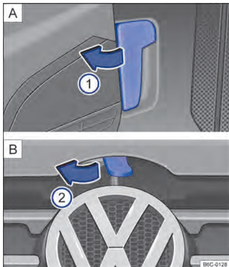
Fig. 181 A Alavanca de destravamento da tampa do compartimento do motor na área para os pés do lado do condutor. B Alavanca de destravamento na parte interna da tampa do compartimento do motor. ▶
