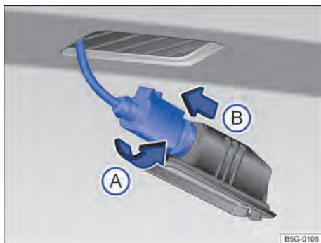
Fig. 171 Lanterna da placa de licença: desinstalar o suporte da lâmpada.
