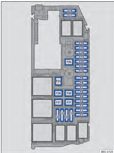
Fig. 175 No compartimento do motor: disposição dos fusíveis.
