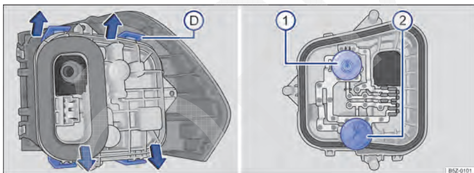
Fig. 178 Lanterna traseira: (D) desinstalar o porta-lâmpadas e (1) e (2) desinstalar as lâmpadas incandescentes.
