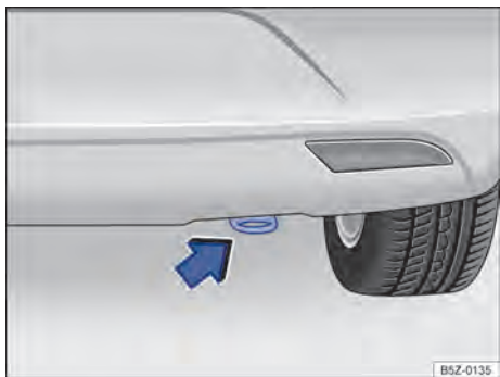
Fig. 189 No para-choque traseiro à direita: argola de reboque.
