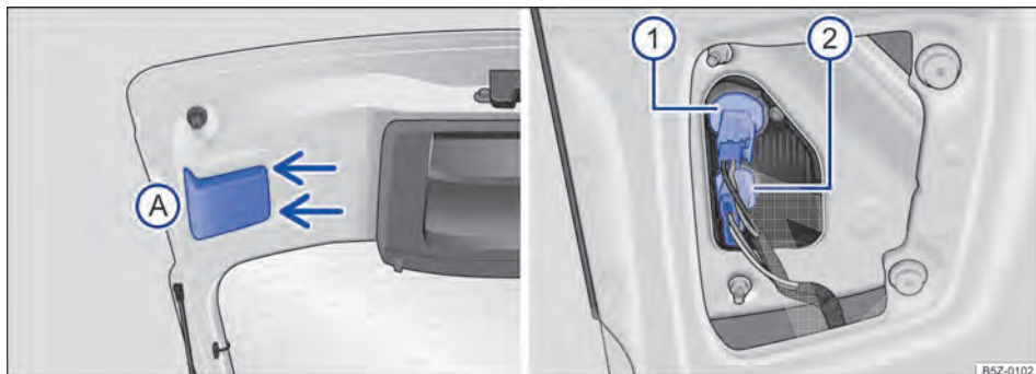
Fig. 179 Lanterna traseira: A desinstalar a cobertura e 1 e 2 desinstalar as lâmpadas.
